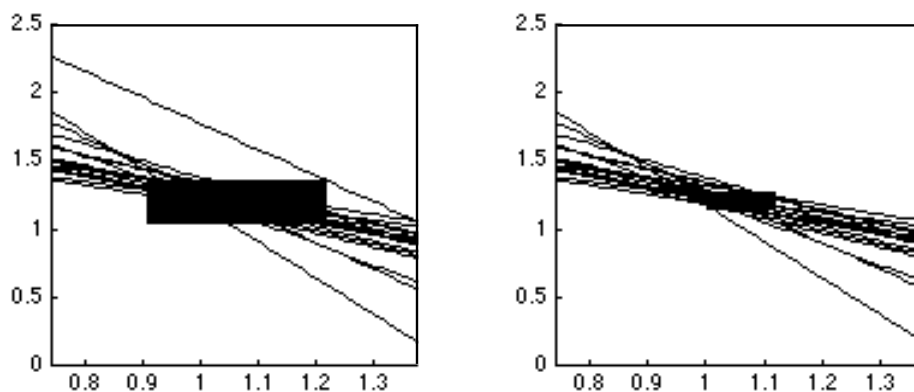
Figure 2a. Caractérisation du modèle incertain dans le plan (\theta_1, \theta_2) avant et après suppression de la mesure aberrante
