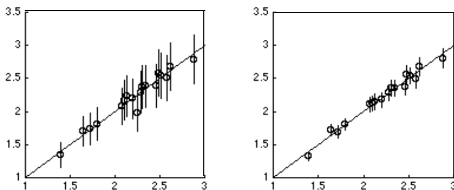
Figure 2b. Caractérisation du modèle dans le plan (mesure-estimation) avant et après détection-suppression de la mesure aberrante.
