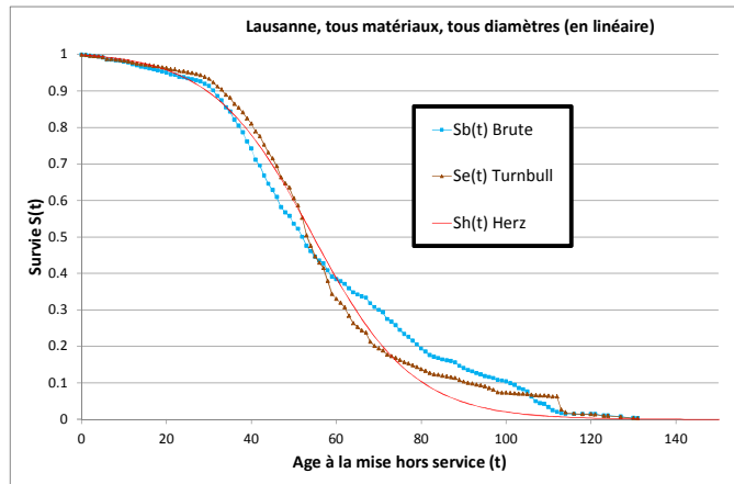
Figure 3. Probabilité pour un mètre linéaire de tronçon de ne pas être mis hors service à un âge supérieur à t (survie) à Lausanne, tous matériaux confondus
