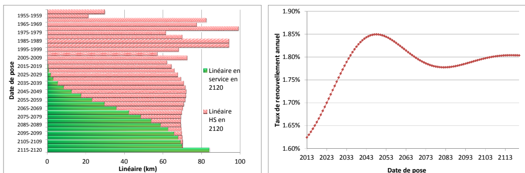
Figure 4 Reconstitution du linéaire passé et prévision des besoins (linéaire, taux de renouvellement) futur jusqu'en 2120 par pas de temps de 5 ans
