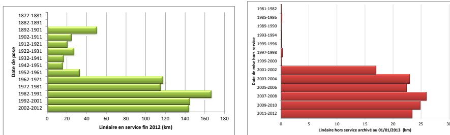
Figure 2. Gauche : Le linéaire en service fin 2012 à Lausanne par décennie de la date de pose. Droite : Le linéaire hors service archivé fin 2012 à Lausanne tous les 2 ans de la date de mise hors service.
