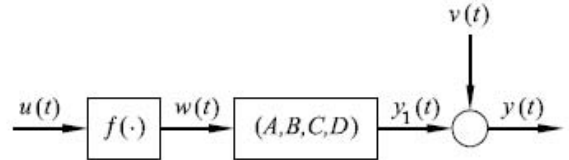
Fig. 2. Hammerstein system.
