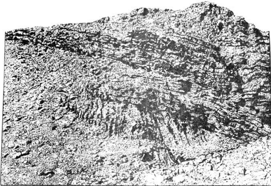
Fig. 8. Discordance des quartzites algonkiens sur l'Archéen au Tizi n'Taratine, Anti-Atlas (d'après Louis Neltner, 1938).
