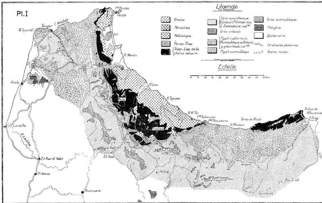
Fig. 12. Schéma géologique d'une partie de la chaîne rifaine située dans la zone du Protectorat espagnol (d'après Paul Fallot et Agustin Marin, 1952).
