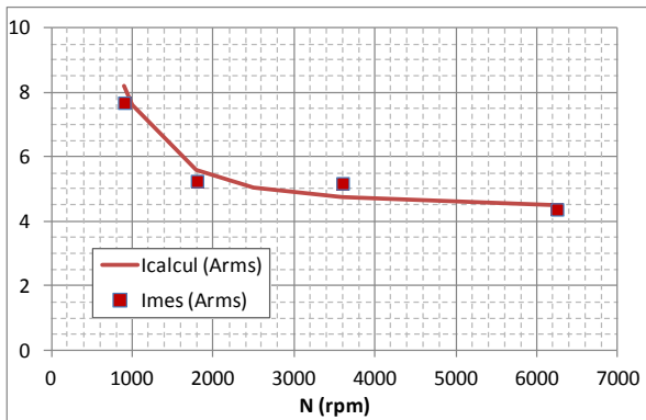
Fig.8: Valeur efficace du courant pour différentes vitesses de rotation, dans le cas où la conversion de puissance est maximale.
