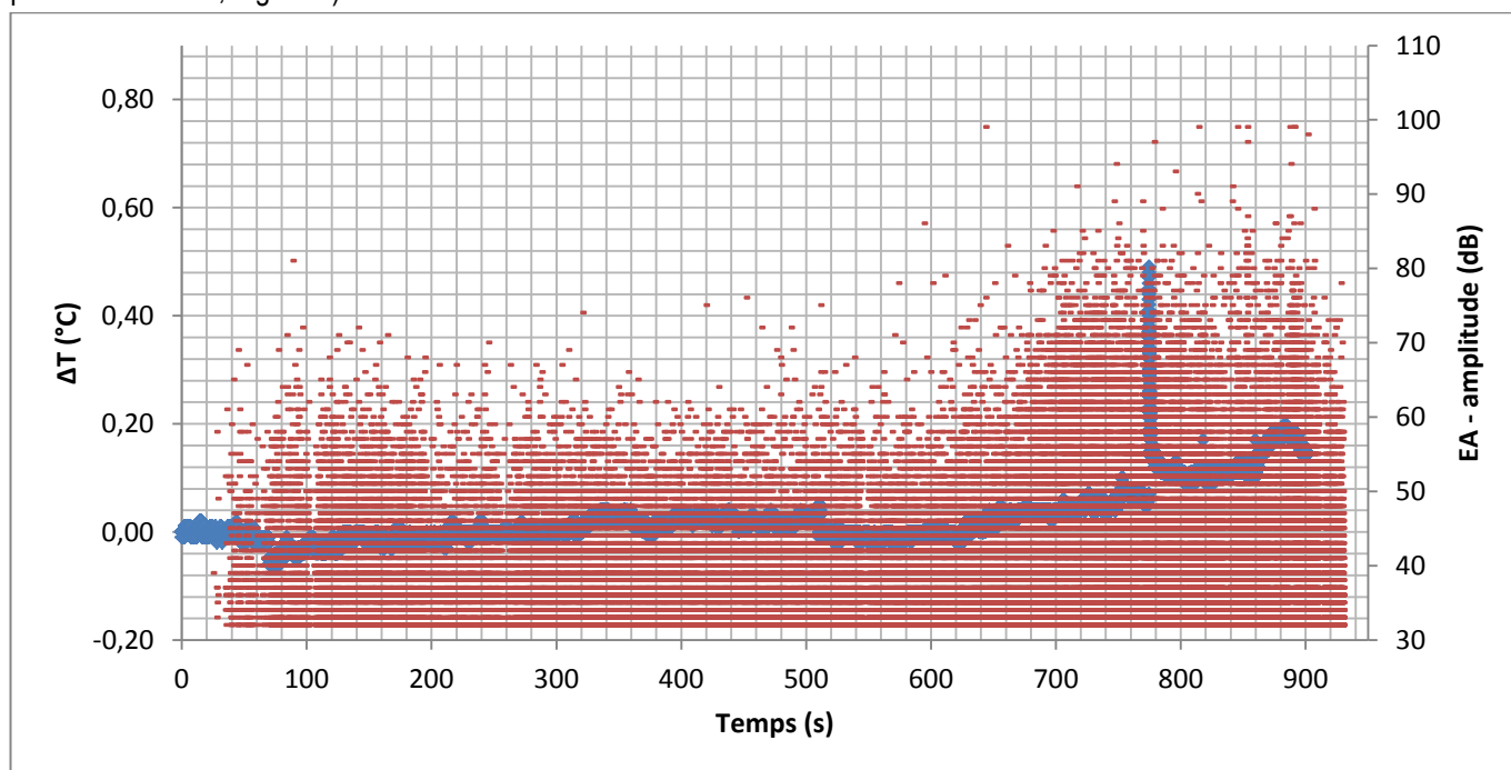
Figure 5. Traction à 0° - Température moyenne et amplitude des événements acoustiques en fonction du temps.
