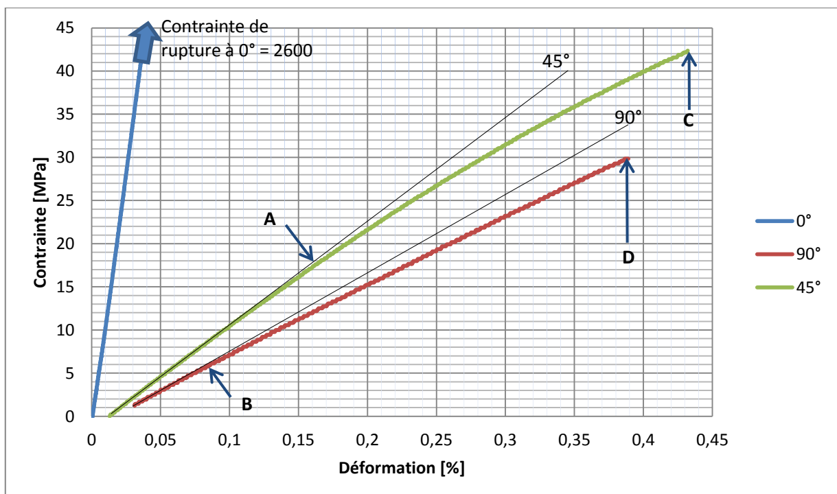
Figure 4. Courbe contrainte-déformation obtenue par les jauges pour les trois directions de fibres
