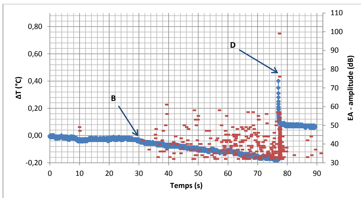
Figure 7. Traction à 90° - Température moyenne et amplitude des événements acoustiques en fonction du temps.
