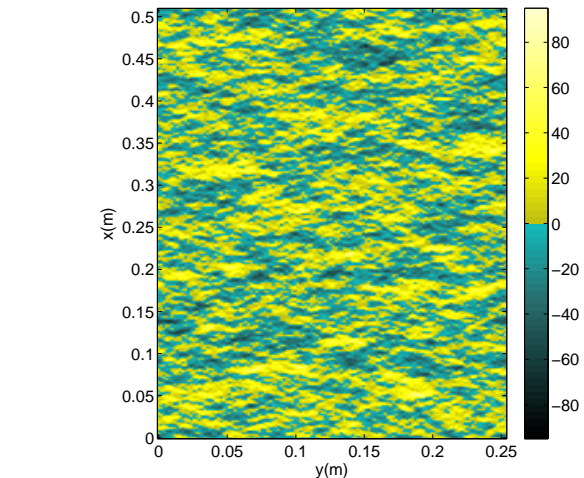
FIGURE 1: Exemple de pression pariétale (en Pa) instantanée synthétisée sur une paroi p_w(x, y, t = t_0)
