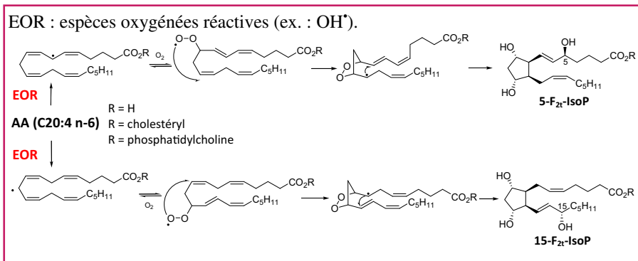
Figure 2 - Mécanisme radicalaire non enzymatique de la formation des isoprostanés. Exemple de la 5- F_{2t} -IsoP et de la 15- F_{2t} -IsoP.
