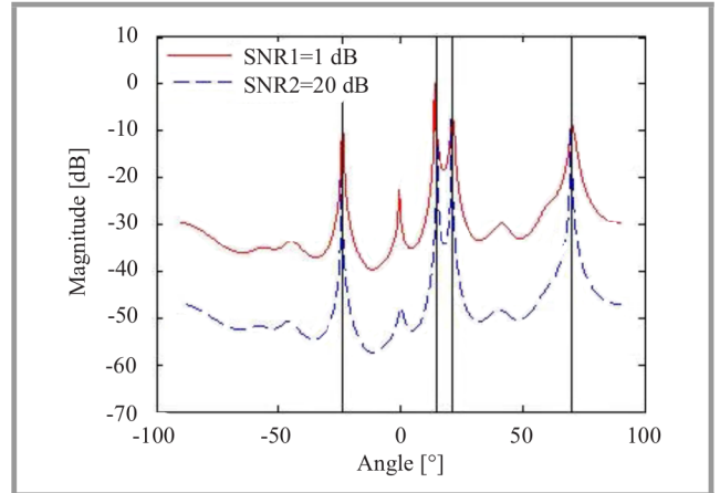
Fig. 9. Propagator spectrum.
