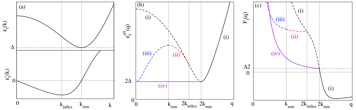
FIGURE 1: Pour la branche d'excitation fermionique de la théorie de BCS à potentiel chimique \mu > 0 , (a) relation de dispersion \epsilon_f(k) et sa dérivée première, utiles à la discussion des branches de stationnarité (12); (b) les branches en question en fonction de q , en trait plein si d'énergie minimale, en tireté sinon; (c) fonction F_f(\check{q}) permettant de minimiser v_f(q) par discussion graphique, voir l'équation (16). Les quantités sur les axes sont adimensionnées comme il est précisé dans le texte.
