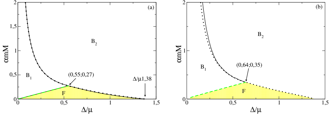
FIGURE 4: (a) Diagramme dans le plan (\check{\Delta} = \Delta/\mu, \alpha = m/M), \mu > 0 , indiquant dans quelle zone la vitesse critique globale v_c^L de l'impureté de masse M a une origine bosonique (cas v_{c,b}^L < v_{c,f}^L , repéré par la lettre B et un fond uni blanc) ou une origine fermionique (cas v_{c,f}^L < v_{c,b}^L , repéré par la lettre F et un fond à rayures jaunes). Le domaine bosonique est séparé en deux sous-domaines B_1 et B_2 par la ligne de transition du premier ordre entre les zones B_0 et B_{q_0} [trait plein noir aux abscisses \check{\Delta} < 0,55 ] de la figure 2b. De façon inattendue, la frontière entre B_2 et F semble coïncider en pratique avec la ligne de transition du premier ordre entre les zones B_{q_{sup}} et B_0 [trait plein noir aux abscisses \check{\Delta} > 0,55 ] de la figure 2b. Autre fait remarquable, la partie non masquée de la ligne de transition du second ordre sur v_{c,f}^L [tireté vert] et la ligne de transition du second ordre entre les zones B_{q_0} et B_{q_{sup}} [tireté noir] sont en pratique indiscernables et situées précisément à la frontière entre B_1 et F . Dernier point notable, la ligne v_{c,f}^L = c [gros pointillé noir] reproduit non seulement la frontière entre B_2 et F , comme il se doit, mais aussi fort bien celle entre B_2 et B_1 . (b) Généralisation du diagramme précédent au cas d'un superfluide d'impuretés bosoniques en mouvement dans le superfluide de fermions, à rapport fixée \mu_B/E_F = 0,1 entre le potentiel chimique des bosons dans le référentiel de leur centre de masse et l'énergie de Fermi. La nouvelle vitesse critique v_c^L présente elle aussi une partition en trois zones, séparées par une discontinuité de sa différentielle seconde (frontière F - B_1 ) ou première (frontières F - B_2 et B_1 - B_2 ) : la zone F (à rayures jaunes), où v_c^L = v_{c,f}^L , et les zones B_1 et B_2 , où v_c^L = v_{c,b}^L . La frontière F - B_1 est très proche de la frontière F_{(i)} - F_{(iv)} à la valeur de \mu_B considérée [tireté vert, interrompu lorsqu'il atteint la zone B_2 ]. La frontière F - B_2 est bien donnée, comme il se doit, par le gros pointillé v_{c,f} = c + c_B , où c ( c_B ) est la vitesse du son dans le superfluide de fermions (bosons), à droite du point triple. La frontière B_1 - B_2 , qui est simplement la frontière B_{q_0} - B_0 à la valeur de \mu_B considérée [trait plein noir], dévie au contraire du pointillé lorsqu'on s'éloigne du point triple sur sa gauche.
