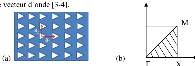
Figure 1 : (a) Exemple d'une structure périodique « cristal phononique » pour des trous triangulaires isocèles. Les vecteurs \mathbf{a}_1 et \mathbf{a}_2 sont les vecteurs périodiques. (b) La première zone de Brillouin et trois points symétriques importants \Gamma(0,0) , X(1,0) et M(1,1) .
