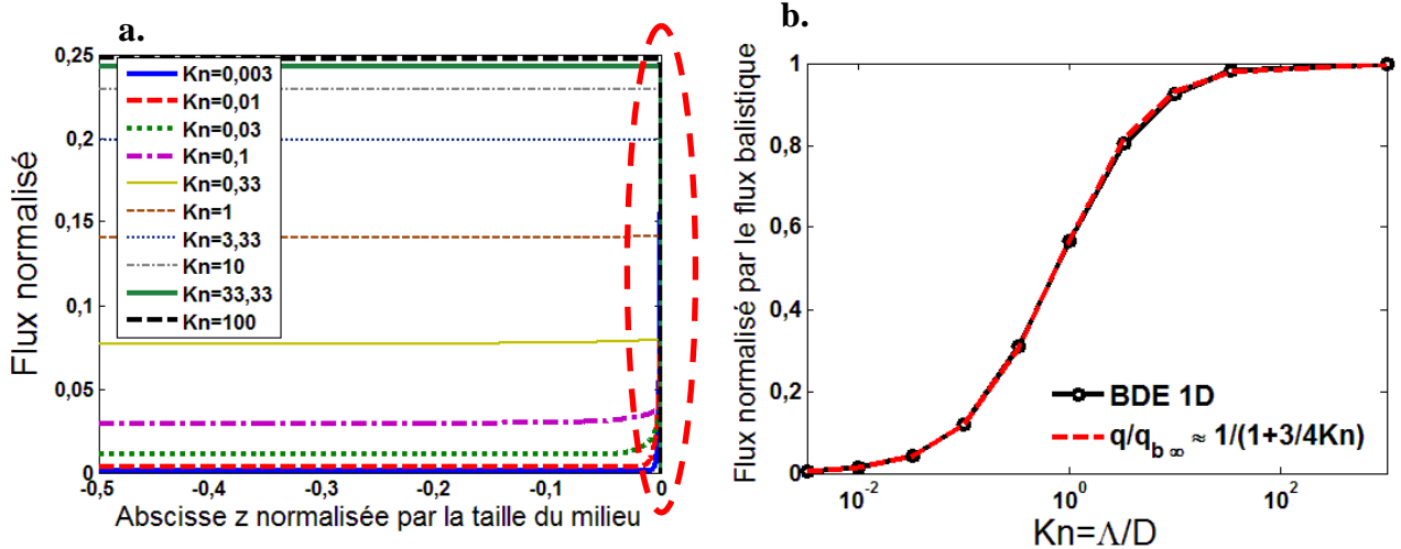
Figure 3 : (a) Profil de flux thermique normalisé par c v \Delta T dans le cas des conditions aux limites asymétriques. Il y a un décalage près de la paroi chaude. (b) Flux thermique normalisé par le flux balistique limite, et comparaison avec l'expression analytique
