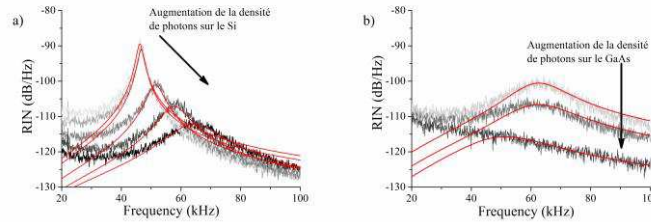
Fig. 1 : a) Spectres de bruit d'intensité relatif pour différentes densités de photons sur le Si. b) spectres obtenus avec une lame de GaAs. Les courbes en rouge représentent les fonctions de transfert théoriques.
