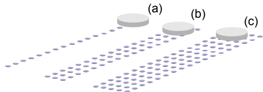
Fig. 4: Simulation scenarios
