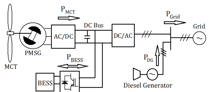
Fig.1 Schéma général d'un système hybride hydrolien/batteries/diesel
