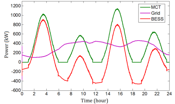
Fig. 9. Puissances transitant dans le système (SoC initial = 0.4).
