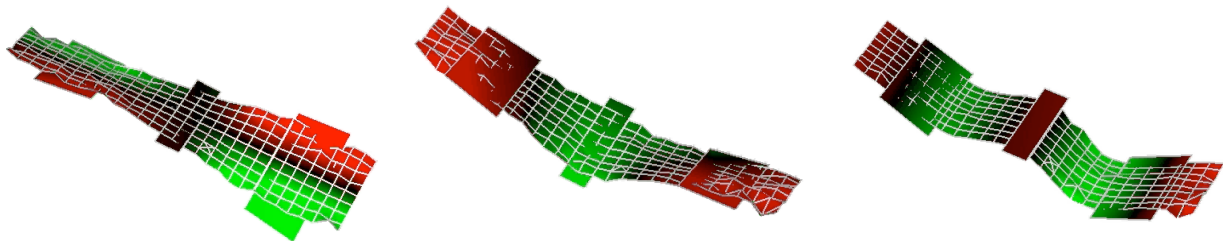
Fig. 4 : Construction expérimentale des trois principaux modes propres sollicitant l'âme en cisaillement. Les trois modes représentés sont torsion antisymétrique (261Hz), Torsion symétrique (279Hz), Cisaillement symétrique (681Hz)
