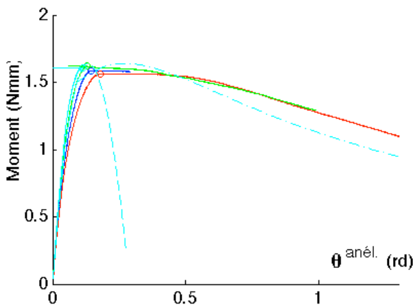
Fig. 21 : Evolution de la rotule plastique
