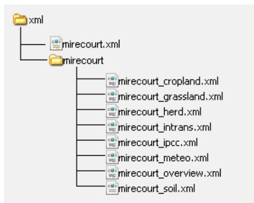
Figure 6 : Exemple d'arborescence de gestion des fichiers de paramétrage du modèle FarmSim
