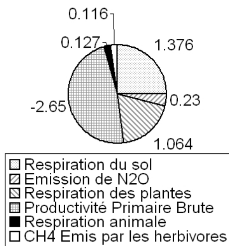
Figure 7 : Bilan des GES simulé pour le cas de la ferme expérimentale de Mirecourt, a) à l'échelle de la parcelle (PaSim) et b) à l'échelle de la ferme (FarmSim)
