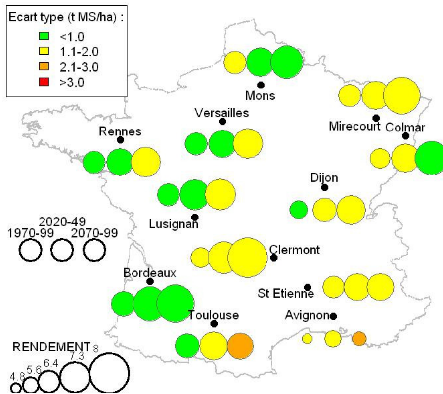
Figure 2 : Evolution du rendement annuel (t MS/ha) pour une prairie permanente intensive implantée sur un sol prairial superficiel, pour les périodes "passé proche" (1970-1999), "futur proche" (2020-2049), "futur lointain" (2070-2099) et pour le scénario climatique A1B,
