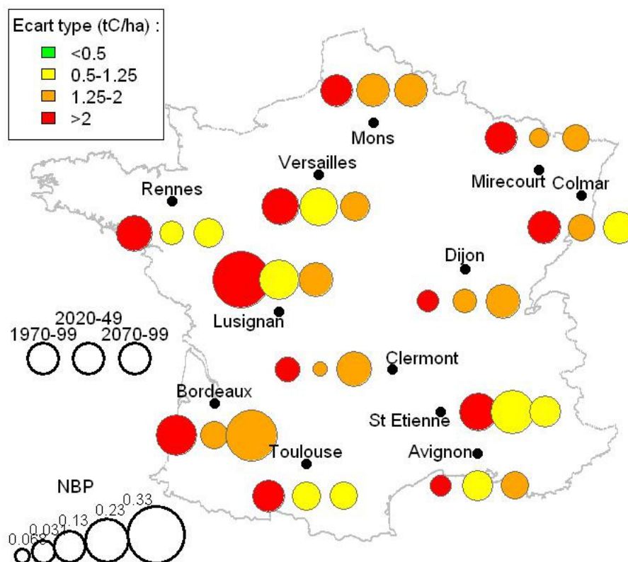
Figure 3 : Evolution du stockage de carbone (Net Biome Productivity, tC/ha/an) pour une prairie permanente intensive implantée sur un sol prairial superficiel, pour les périodes "passé proche" (1970-1999), "futur proche" (2020-2049), "futur lointain" (2070-2099) pour le scénario climatique A1B. Une valeur positive indique une activité de stockage de carbone par les prairies.
