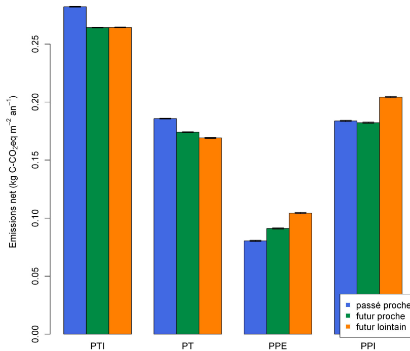
Figure 4 : Emission net de gaz à effet de serre à Avignon pour le scénario A2 (réchauffement de 4°C à la fin du siècle) pour une prairie implantée sur un sol superficiel, pour les périodes "passé proche" (1970-1999), "futur proche" (2020-2049), "futur lointain" (2070-2099) et pour différentes gestions : PTI (Prairie temporaire de ray-grass Irriguée), PT (Prairie temporaire de ray-grass pluviale), PPE (Prairie Permanente Extensive), PPI (Prairie Permanente Intensive)
