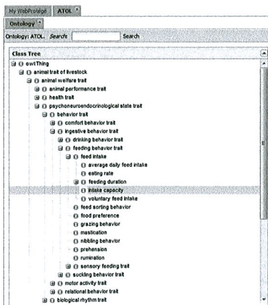
Figure 1 - Structure hiérarchique de l'ontologie ATOL, avec les sept finalités d'intérêt à la racine (A), et l'arborescence de la finalité «Bien-Etre» ( animal welfare trait ) aboutissant par exemple au caractère unitaire mesurable «capacité d'ingestion» ( intake capacity ) (B).
