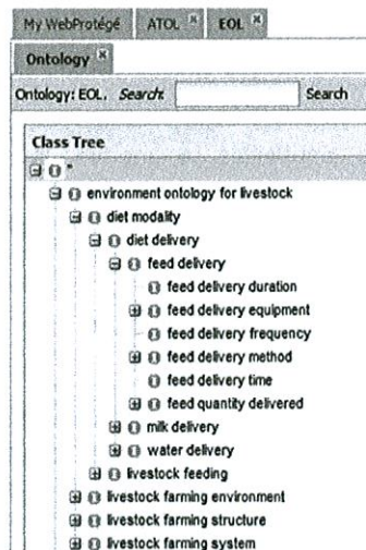
Figure 2 - Structure hiérarchique de l'ontologie EOL.
