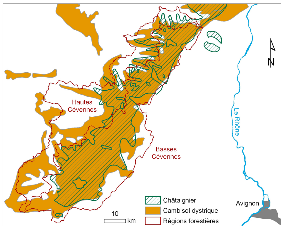
Carte 4 : Aire de distribution du Châtaignier et étendue des Cambisols dystriques dans les Cévennes.
