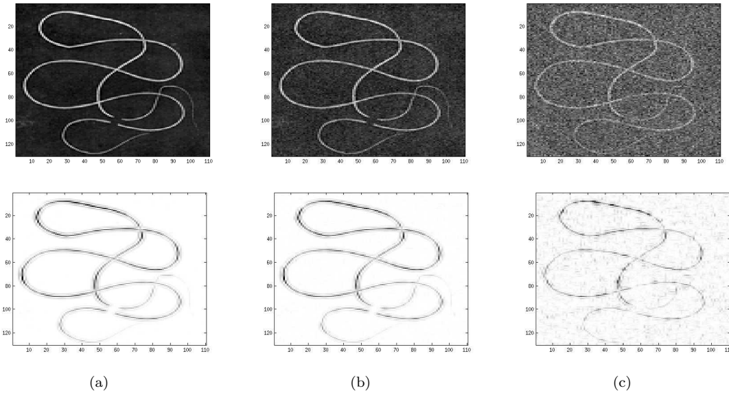
Figure 1. Robustness of the topological gradient with respect to noise on a synthesis image using (16), (a) : Image without noise, (b) : Noisy image with Gaussian noise, PSNR=26dB, (c) : Noisy image with Gaussian noise, PSNR=14dB, top : Initial image, down : Topological gradient using (16), Robustesse du gradient topologique par rapport au bruit pour une image synthétique en utilisant (16), (a) : Image sans bruit, (b) : Image bruitée par du bruit Gaussien, PSNR=26dB, (c) : Image bruitée par du bruit Gaussien, PSNR=14dB, en haut : Image initiale, en bas : Gradient topologique utilisant (16)
