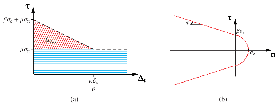
Fig. 4 – (a) Contrainte de cisaillement fonction du déplacement tangentiel pour une fissuration en mode II et (b) surface de rupture
