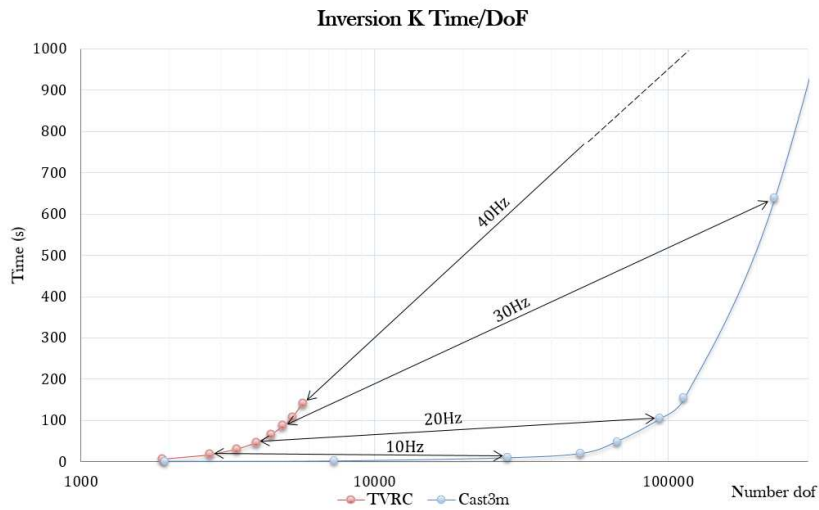
Figure 10. Comparaison des temps de calcul EF et TVRC
