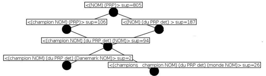
FIG. 2 – Extrait du diagramme de Hasse contenant des motifs séquentiels.
