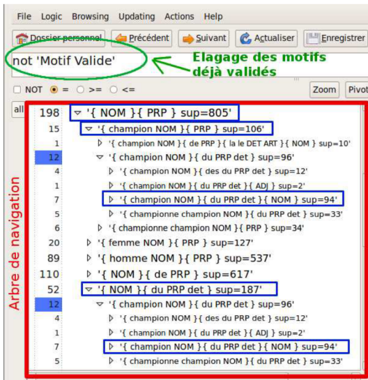
FIG. 1 – Navigation dans les patrons linguistiques pour les valider.
