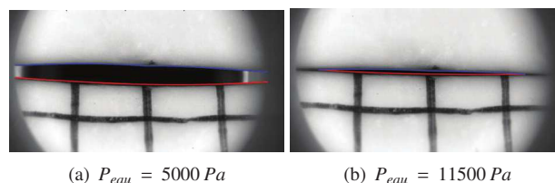
FIGURE 8 – Détection de contours de l'air glottique pour la mesure du gonflement des maquettes de plis vocaux soumis à une pression d'eau P_{eau}
