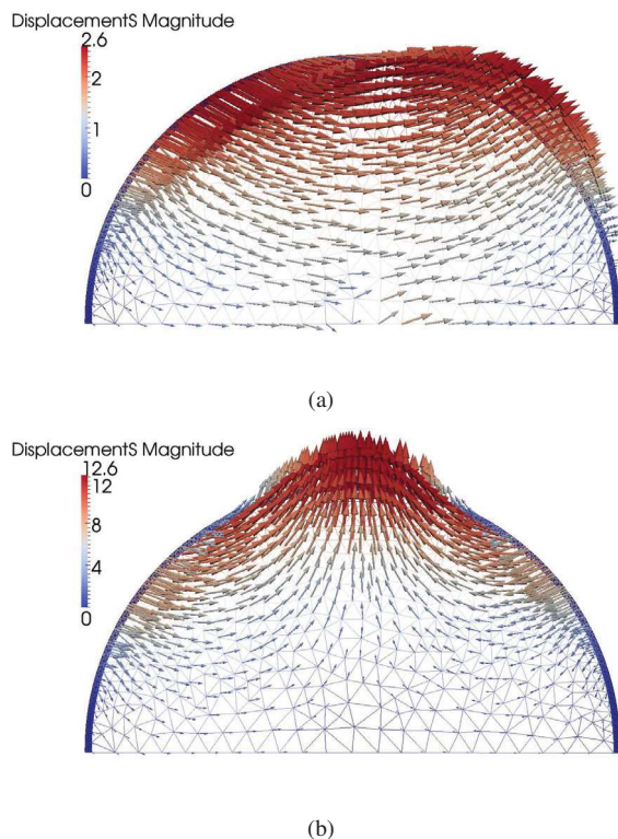
FIGURE 7 – Déformée modale en déplacement des 1 er et 3 em mode de vibration hydro-élastique
