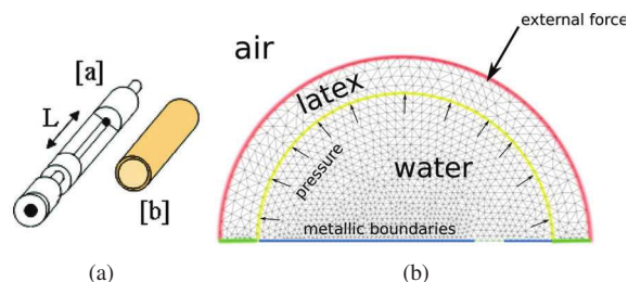
FIGURE 2 – Maquette des plis vocaux (a) et géométrie des domaines couplés (b)
