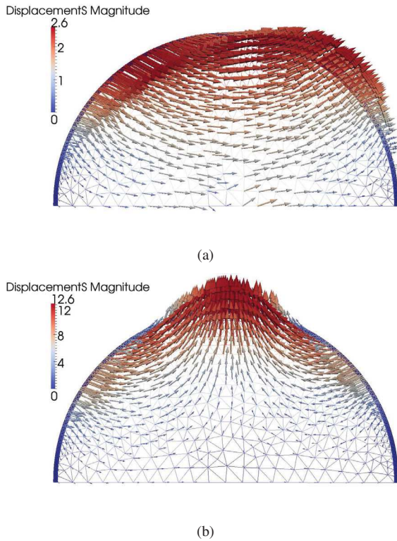
FIGURE 7 – Déformée modale en déplacement des 1 er et 3 me mode de vibration hydro-élastique
