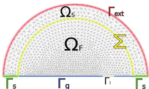
FIGURE 3 – Domaines et interfaces du problème couplé
