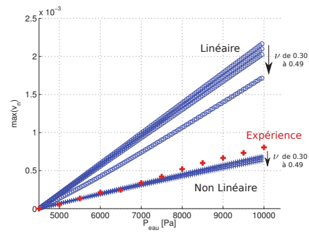
FIGURE 9 – Déplacement statique maximal du latex sous l’action de la pression d’eau P_{eau}
