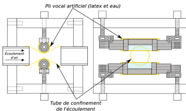
FIGURE 1 – Vues latérale (à gauche) et axiale (à droite) de la maquette [10].
