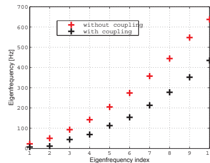
FIGURE 6 – Les dix premières fréquences de résonance du modèle 2D avec (noir) et sans (rouge) prise en compte du couplage hydro-élastique
