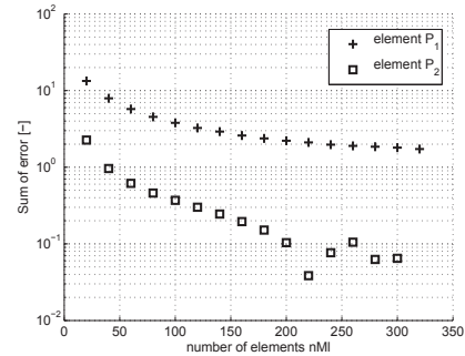
FIGURE 5 – Somme de l'erreur sur les dix premières fréquences propres en fonction du nombre d'éléments nMI (b)
