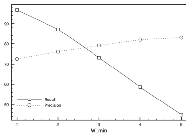
(d) Précision et rappel des motifs LSR en fonction de W_{min} ( minconf = 0.6 , N_R = 5 )
