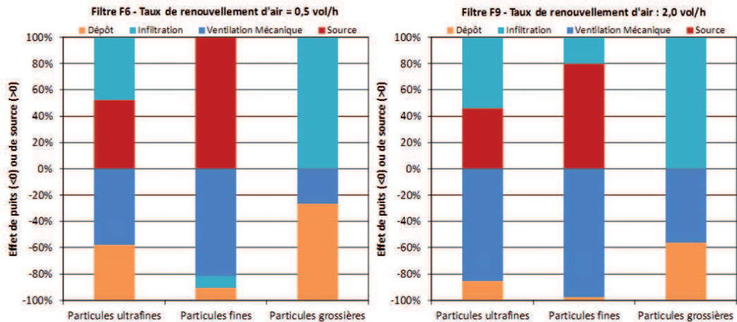
Figure 16 : Contributions du dépôt, de l'infiltration, de la ventilation mécanique et de la source à l'équilibre de la concentration intérieure en particules de l'ambiance pour deux types de filtres et de renouvellement d'air.
