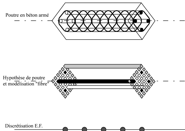
Figure 1 : Principe d'une poutre multifibre.
