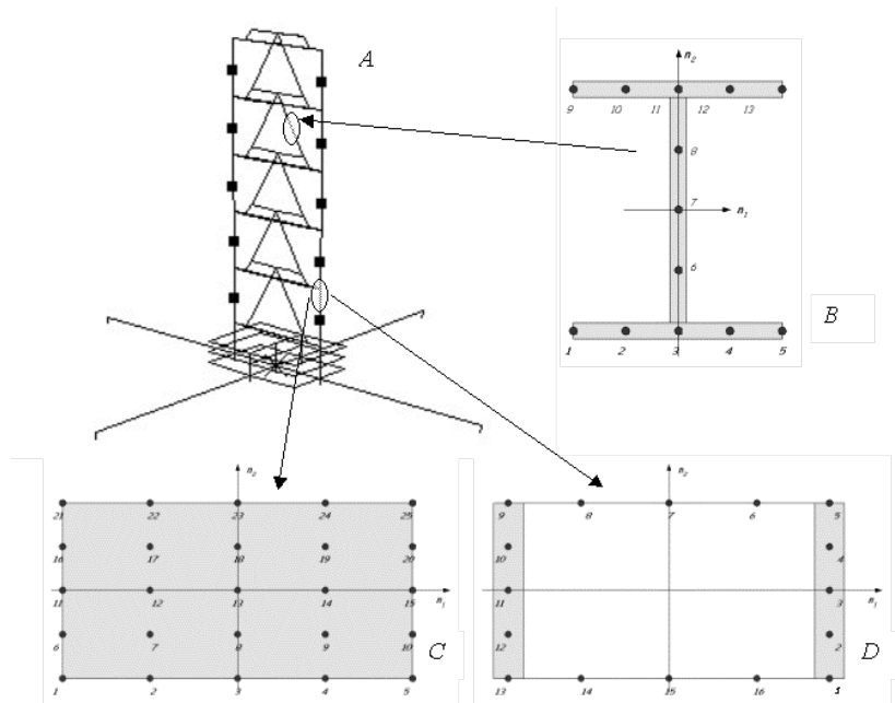
Figure 3 : A) Maillage de la structure B) Section adoptée pour le système de contreventement C) Eléments de section rectangulaire pour le béton D) Eléments de section de type « box » pour les armatures et les masses aux différents étages. La position et le nombre des points d'intégration sont aussi indiqués.
