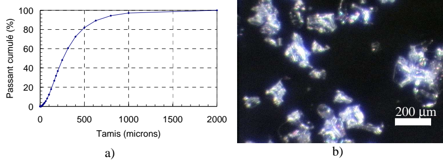
Figure 1. Distribution granulométrique des éléments fins (0-2mm) des déchets de mousse de PUR (a) et visualisation par vidéomicroscopie (b)
