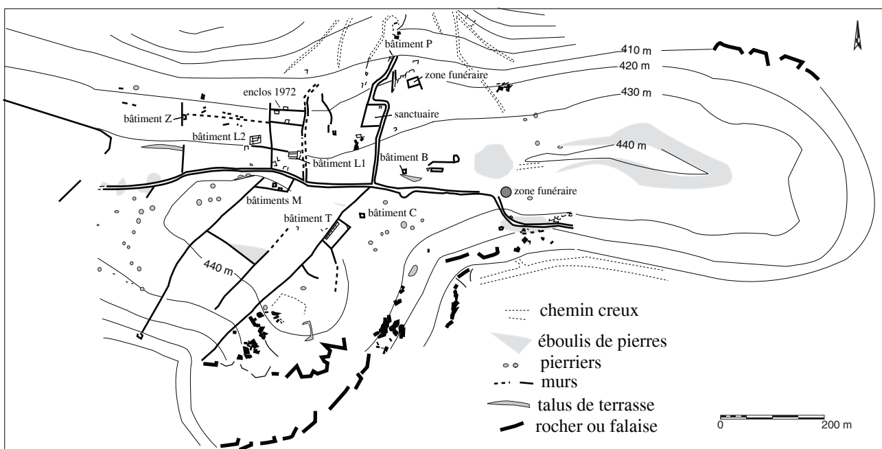
+ Fig. 6. Plan du site du Wasserwald à Haegen (57) d'après Pétry 1977, fig. 3 et Pétry 1994, p. 1. Relevé Ensai et E. Kern.
