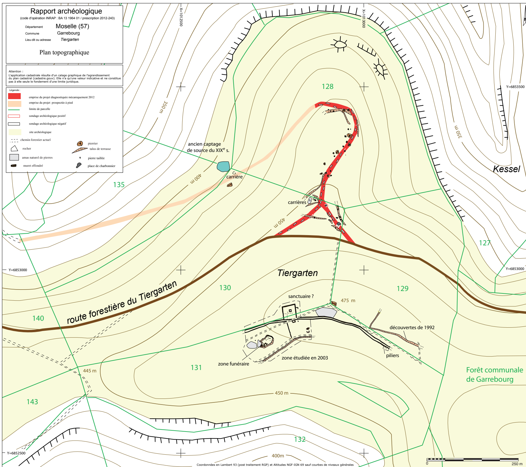
+ Fig. 10. Plan d'une partie du hameau du Tiergarten-Ditchelkopf à Garrebourg (57) relevé lors d'une opération préventive (Forelle, Meyer 2013a).
