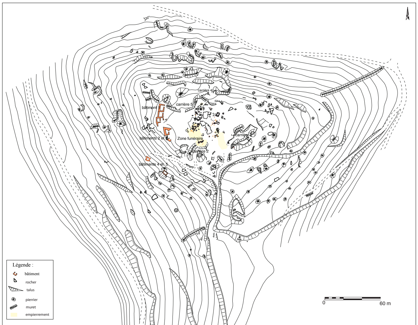
+ Fig. 7. Plan du site de la Croix-Guillaume à Saint-Quirin (57). Foudilles 1994-1999.
