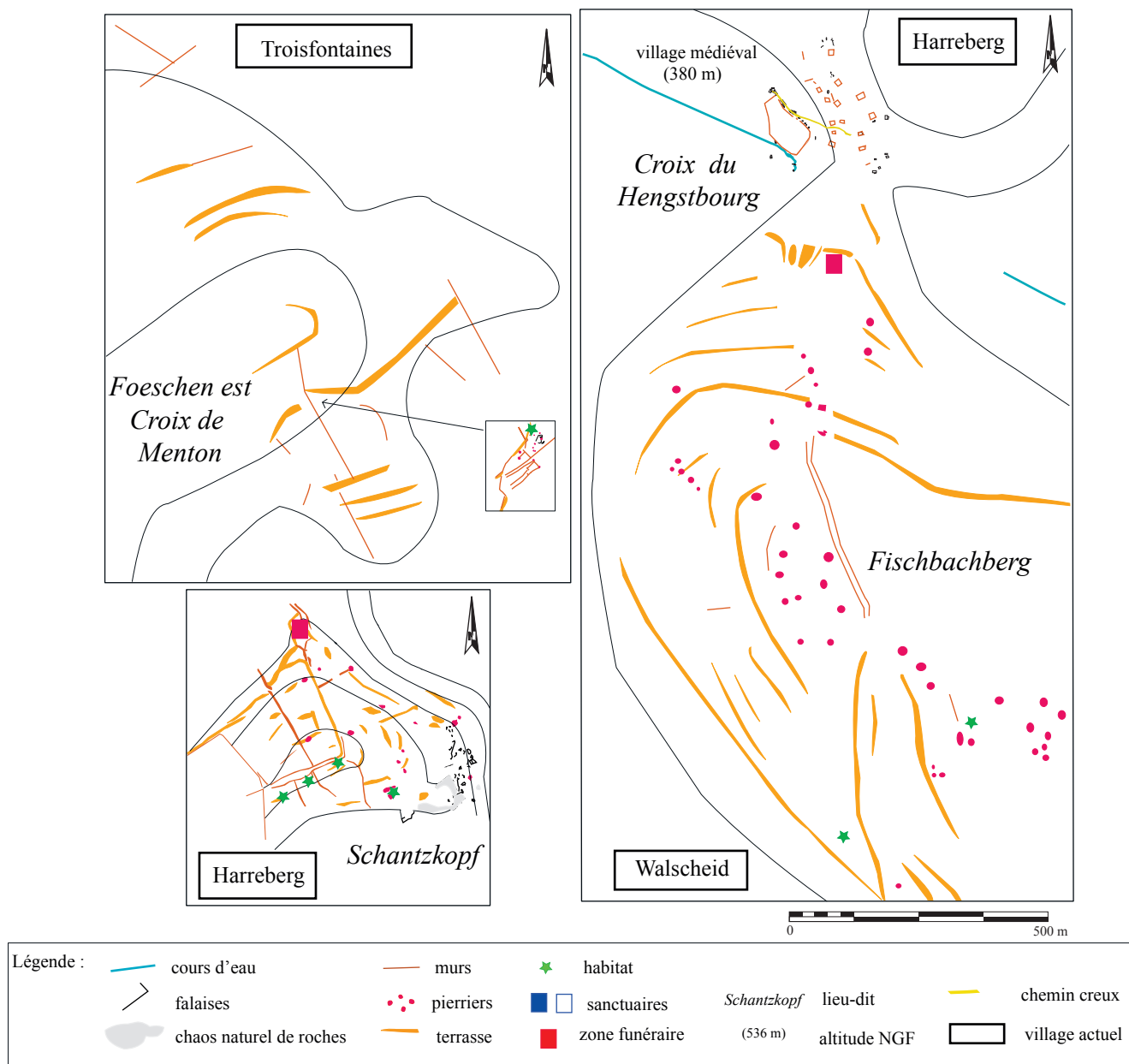
+ Fig. 24. Plans des structures agraires et parcellaires fossiles des secteurs de Troisfontaines Foeschen , nord (57), d'après les relevés du R. P. Goester (1952), de Harreberg Schantzkopf (57) et de Walscheid Fischbachberg (57) d'après Courtney Edward Stevens (1937).
