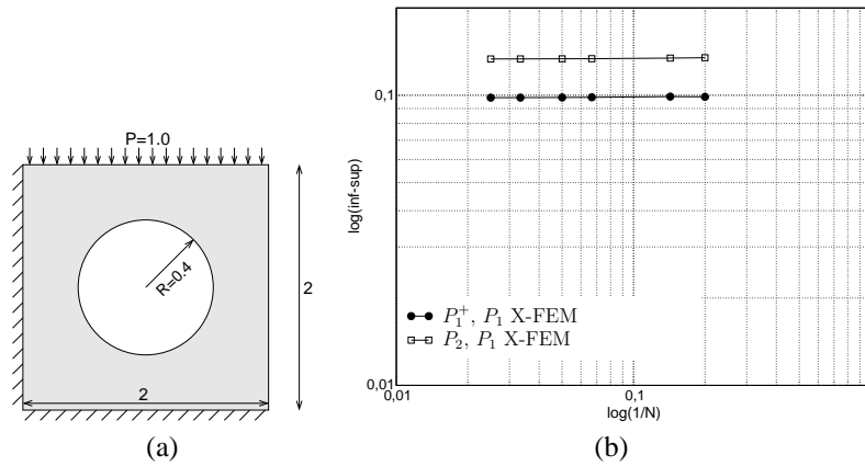
Figure 4. Évaluation du inf-sup pour les trous : (a) problème de référence, (b) Évolution du inf-sup numérique.
