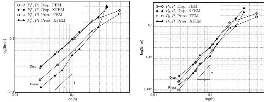
Figure 3. Étude de convergence, plaque incompressible avec un trou. Gauche : Mini, Droite : T6T3.
