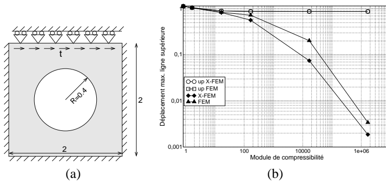
Figure 5. (a) Problème de cavité, (b) Évolution du déplacement sur la ligne supérieure en fonction du module de compressibilité.
