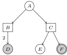
Fig. 1. Game \mathcal{G} .
