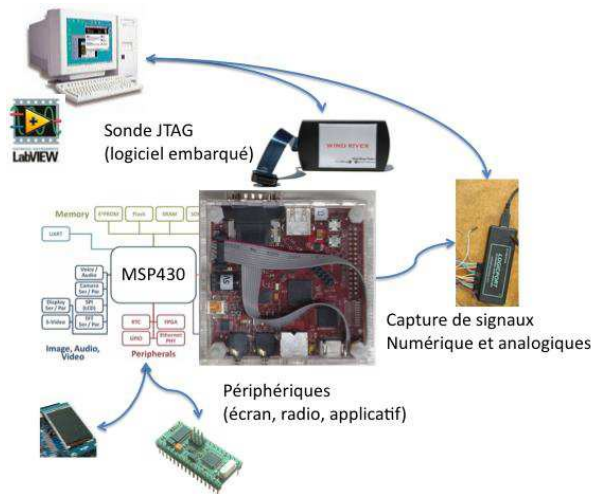
Fig 7 : Synoptique d'accès à distance des ressources
