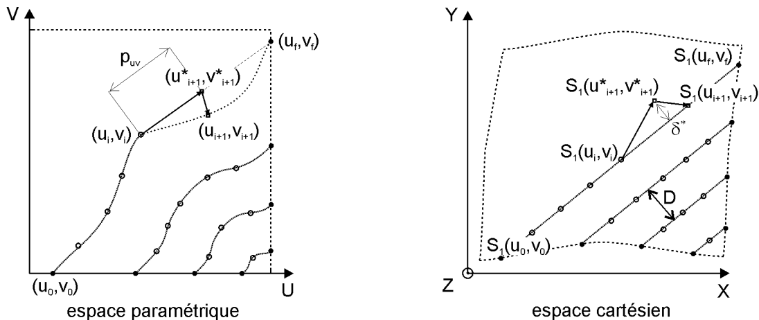
Fig. 4 : Calcul des positions de l'outil
