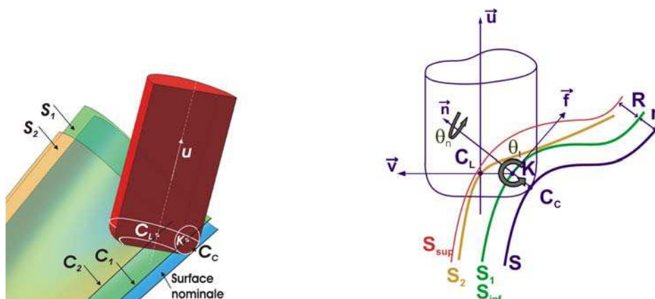
Fig. 2 : Modèle d'usinage surfacique en 5 axes
