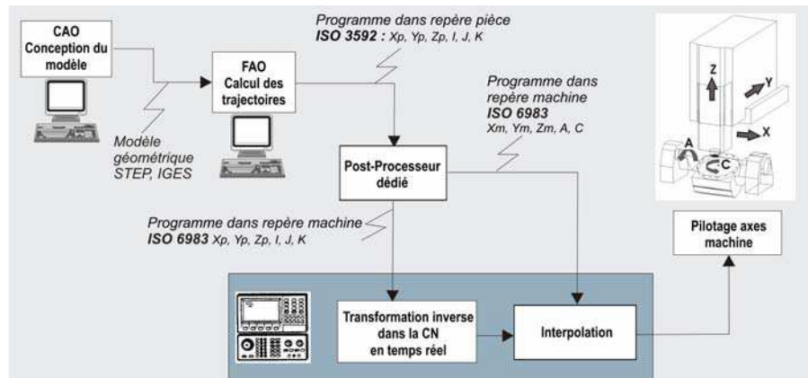
Fig. 1 : Chaîne numérique en 5 axes
