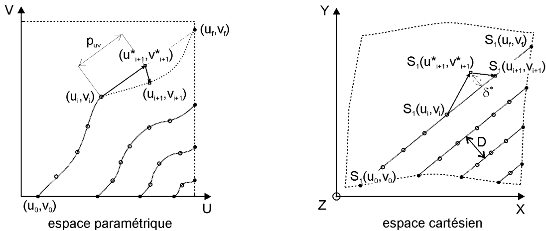
Fig. 4 : Calcul des positions de l'outil
