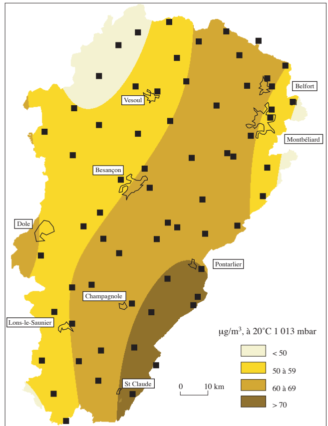
Fig. 2 - Tendances régionales de l'ozone du 2 mai au 3 juin 2002
