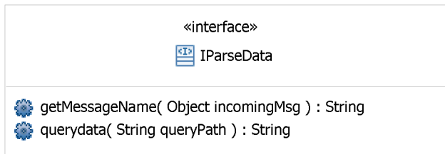
Fig. 3. ParseData Interface of RV4WS
