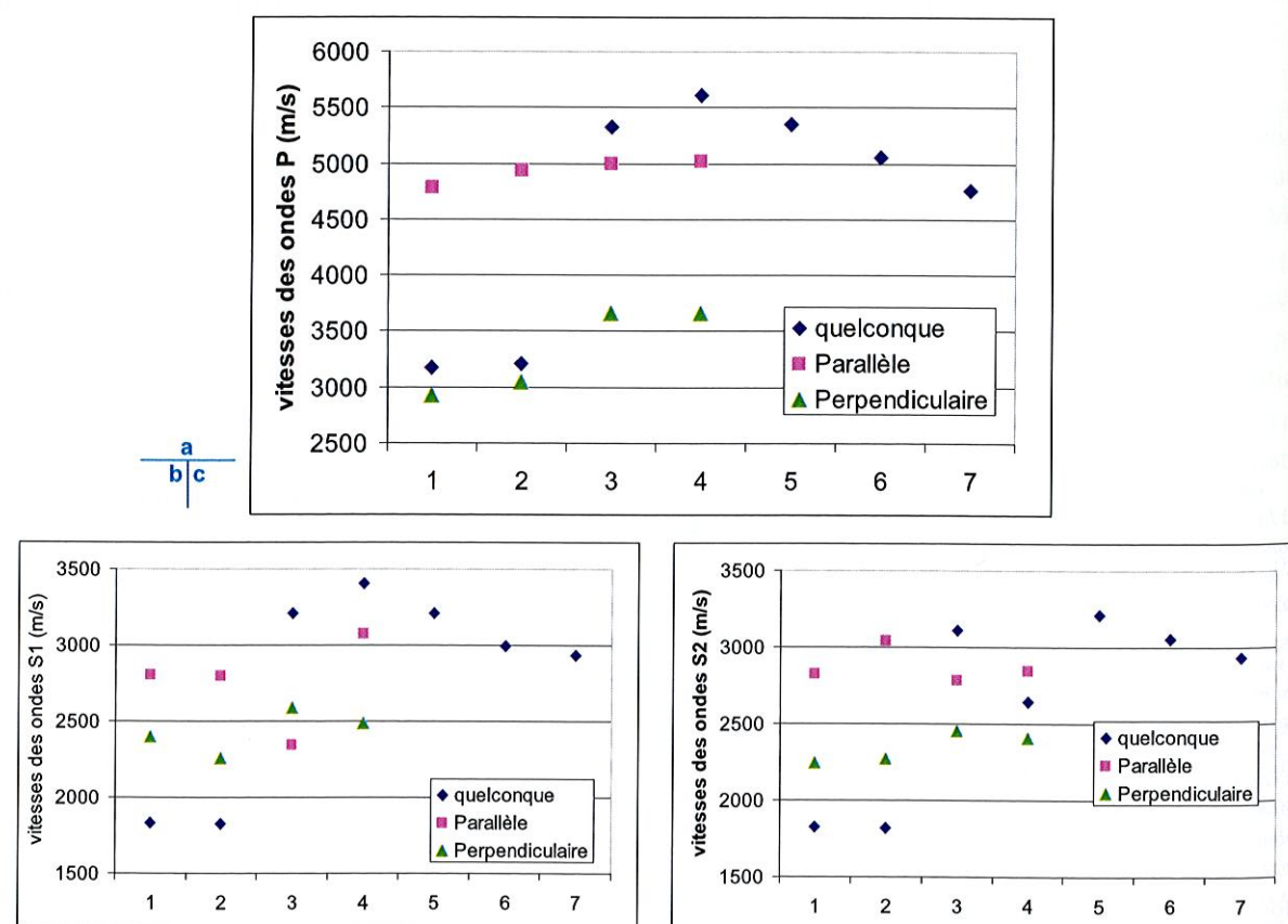
figure 9 Vitesse des ondes P (a), S1 (b) et S2 (c) en fonction de l'orientation de la foliation de la roche par rapport à l'axe de la carotte.
