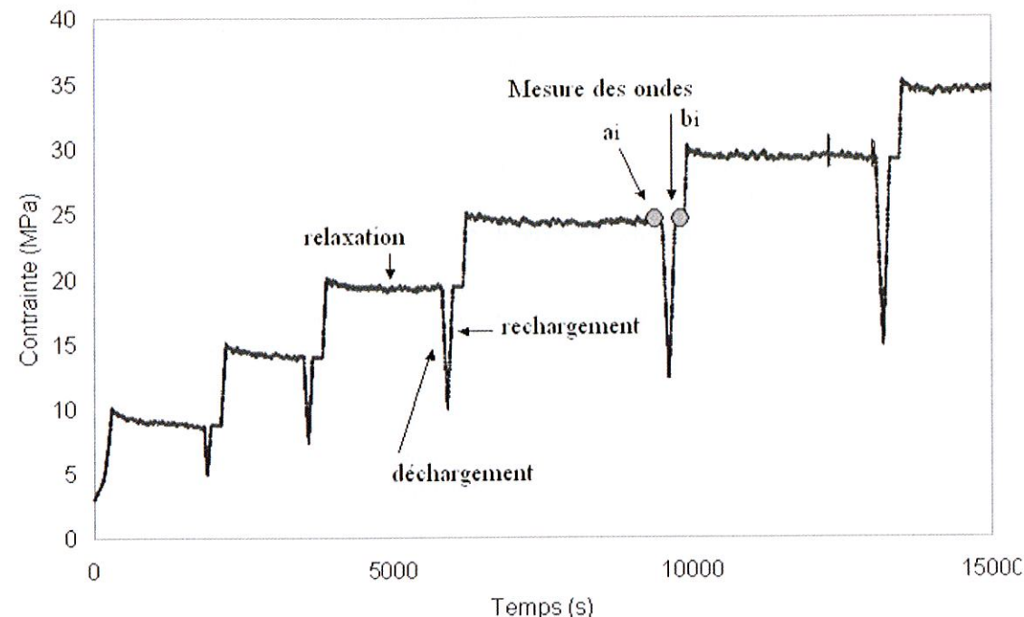
figure 2 Historique du chargement et points de mesure de la vitesse des ondes élastiques (a, b, avec i numéro du cycle) – éprouvette R640.
