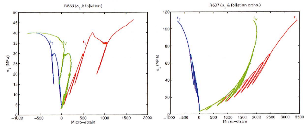
figure 7 Courbes contrainte-déformation issues des compressions uniaxiales de R633 (à gauche, foliation sub-parallèle à \sigma_1 ) et R637 (à droite, foliation sub-orthogonale à \sigma_1 ). Les déformations longitudinales ( \epsilon_x ) sont en rouge, les déformations transversales ( \epsilon_y ) en bleu, et les déformations volumiques ( \epsilon_v ) en vert, d'après Wassermann et al. (2009a).
