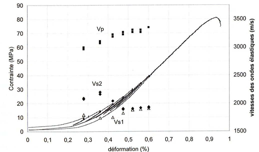
figure 5 Courbe contrainte-déformation caractéristique des essais uniaxiaux avec mesures des vitesses et enregistrement des événements d'EA sur 4 capteurs. L'éprouvette (R 640) est carottée perpendiculairement au plan de foliation.
