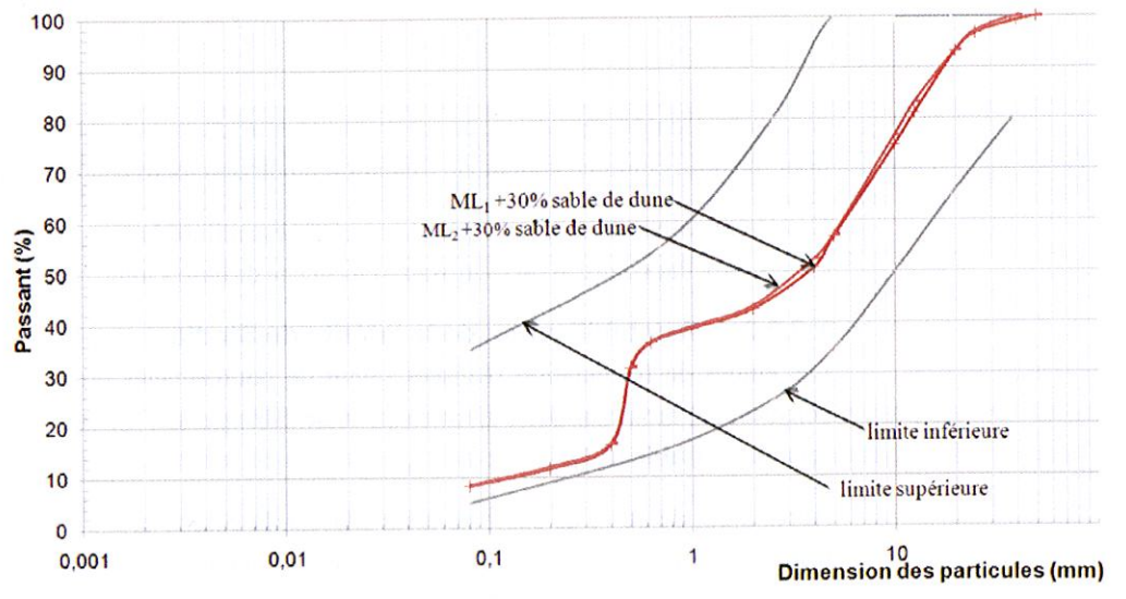
figure 5 Représentation des courbes granulométriques de ML 1 + 30 % de sable et ML 2 + 30 % de sable et du fuseau granulométrique du CEBTP (1972) pour une utilisation en couche de fondation de route à faible trafic.
