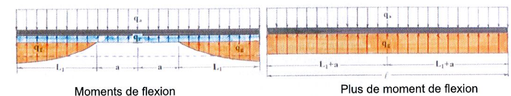
figure 24 Équilibre des charges et pressions du sol sur une poutre horizontale.
