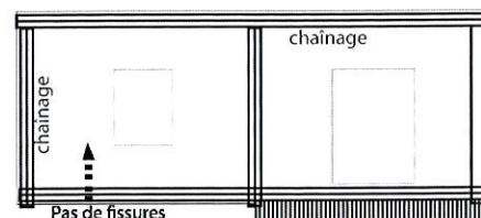
c. Disposition des chaînages
