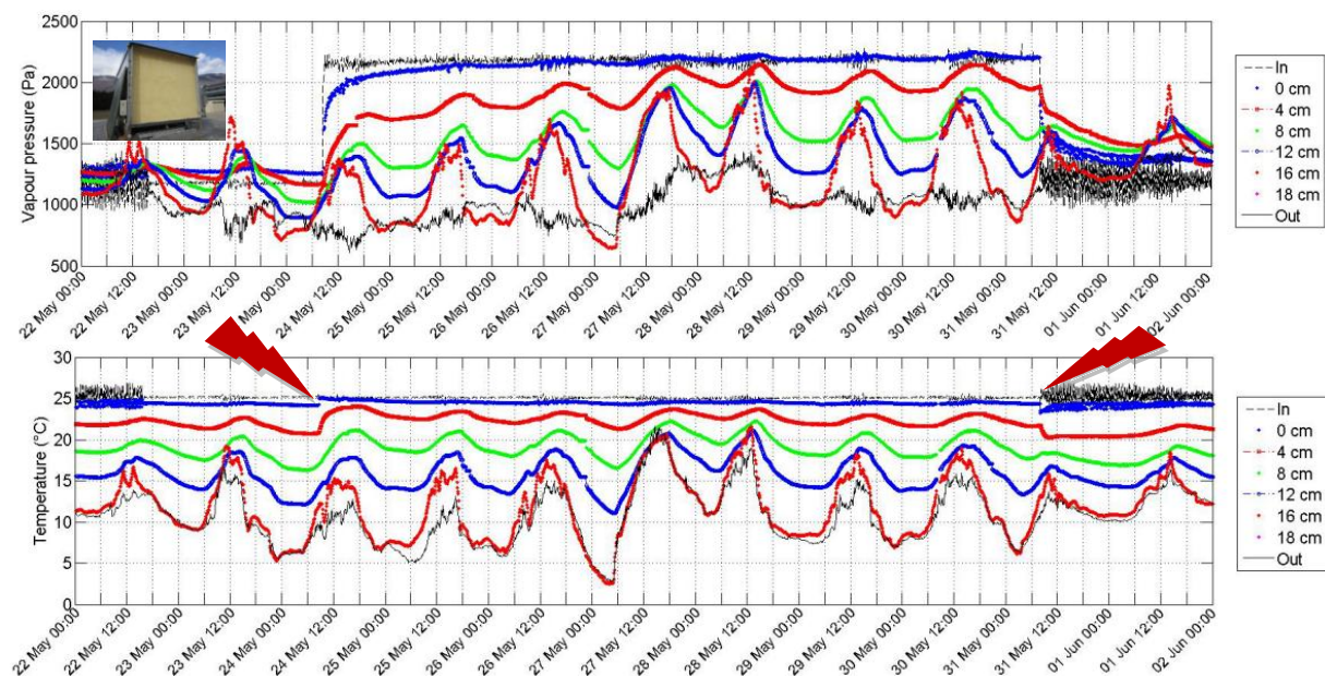
Figure 4. Evolution des pressions partielles de vapeur et des températures à différentes profondeurs dans la paroi n°3 (16cm de fibre de bois + enduit extérieur) sur la cellule Passys, soumise au climat naturel à l'extérieur et à un échelon d'humidité à l'intérieur.
