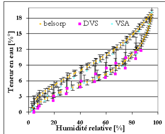
Figure 1. Isothermes de sorption-désorption de l'isolant de fibre en bois à 20°C, obtenues par différentes méthodes au LASIE
