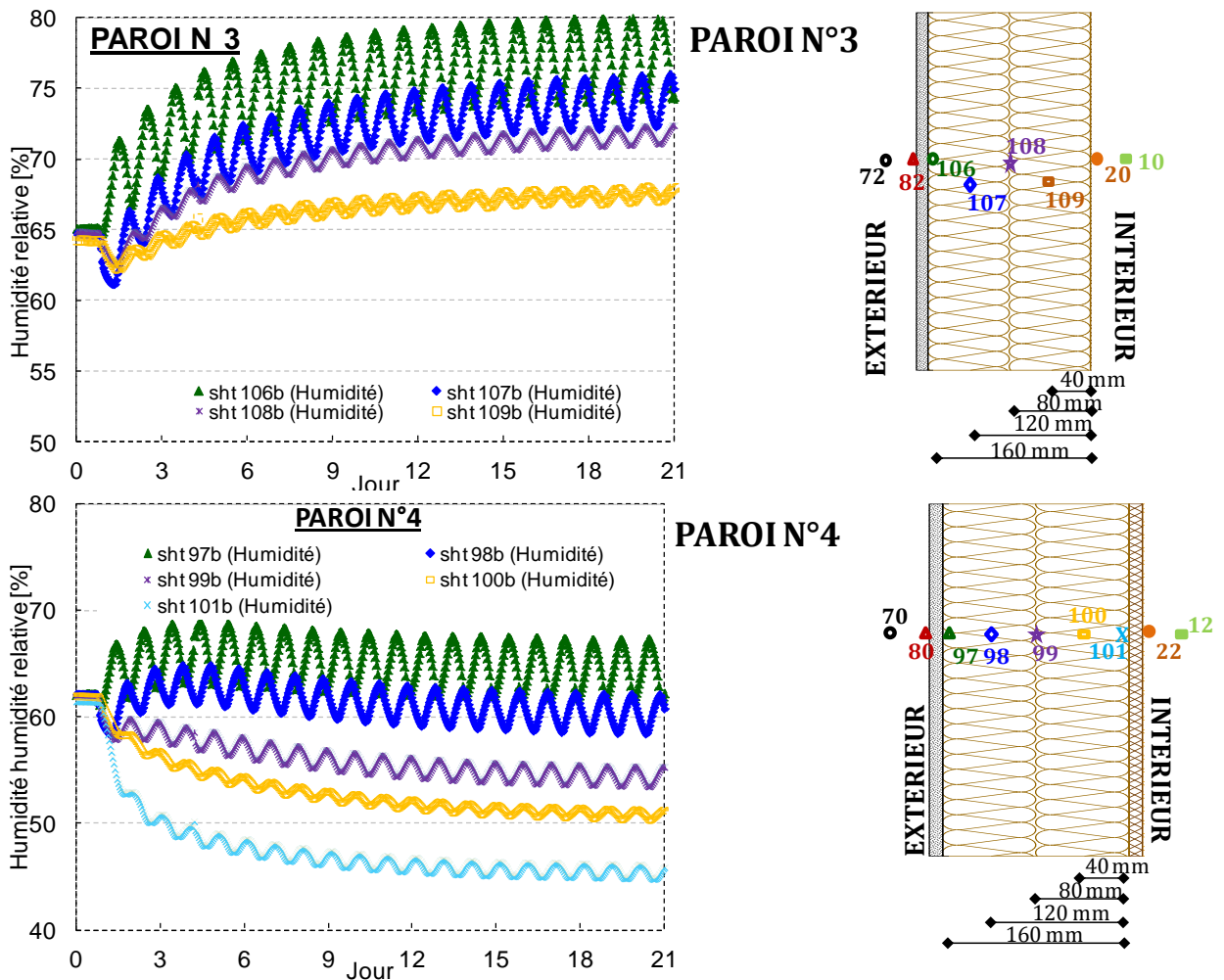
Figure 3. Evolution temporelle des profils de température et d'humidité relative de l'air dans les parois avec la fibre de bois seule (N° 2), protégé par l'enduit extérieur (N°3) et protégé par l'enduit extérieur et OSB (N°4), soumise à des conditions climatiques oscillantes.
