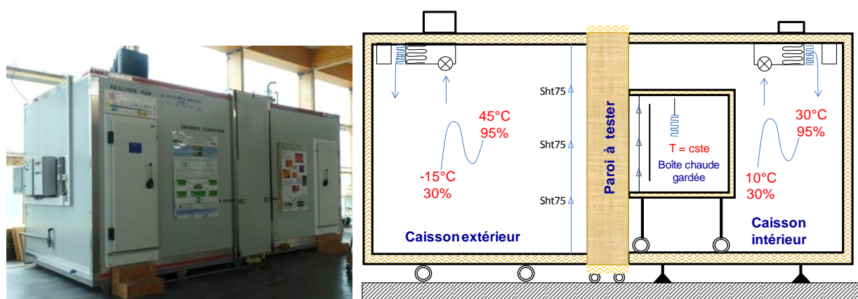
Figure 2. Photo et schéma de principe de la double enceinte climatique du LERMAB
