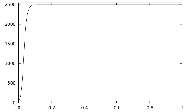
(d) Mean centroid evolution
