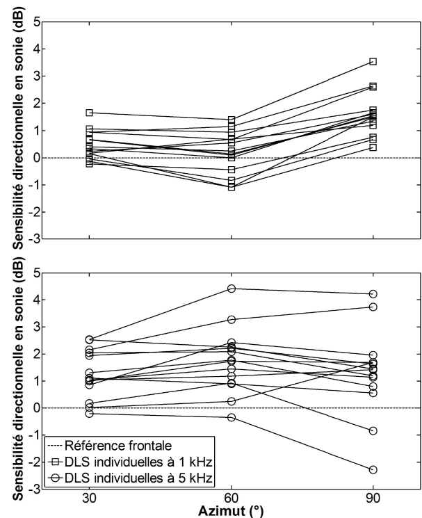
FIGURE 1 – Sensibilités directionnelles en sonie (DLS) à 30, 60 et 90° d'azimut, mesurées pour chacun des 14 auditeurs, dans le cas d'une simple source de bruit à bande étroite centrée à 1 kHz (en haut) ou 5 kHz (en bas).
