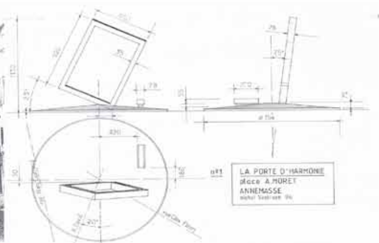
Plans et coupes de l'oeuvre. Documents extraits du dossier de présentation du projet
