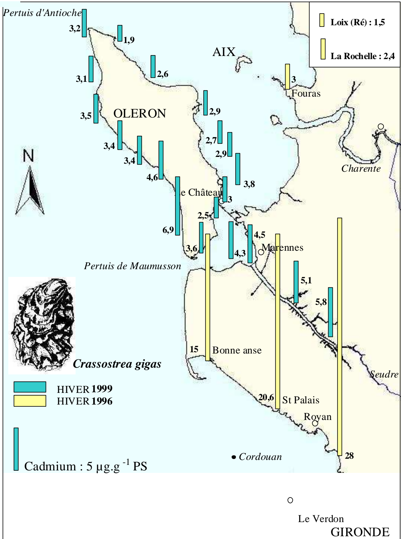
Figure 3 : Concentrations en Cd (µg/g de poids sec) dans les tissus des huîtres sauvages Crassostrea gigas prélevées le long des côtes de Charente-Maritime.
