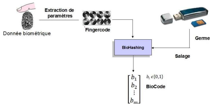
Figure 2: Schéma de BioHashing
