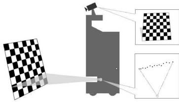
FIGURE 1 – Illustration du processus d'étalonnage caméra-téléporteur utilisant une mire plane. Le système d'acquisition, ici un robot, perçoit par son télémètre un plan et la caméra détecte le damier. Les deux informations sont intégrées au sein d'une fonction objectif tandis qu'un algorithme de minimisation retrouve le paramétrage extrinsèque du système.
