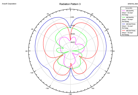
Figure 3b. exemple de diagrammes de rayonnement théoriques à 5.26 GHz.
