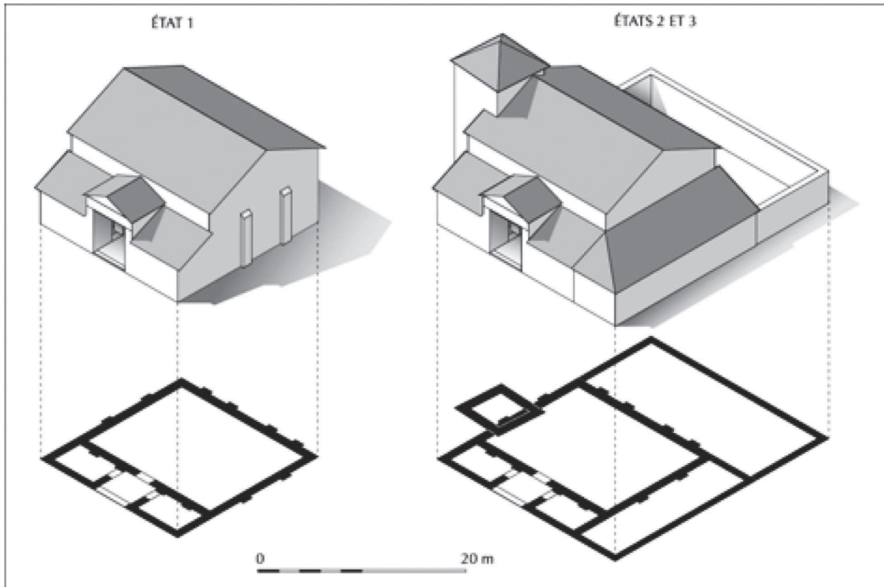
Proposition de restitution par état des volumes du bâtiment 2 de Chaucenne(Doubs) (dessin C. Gaston).
