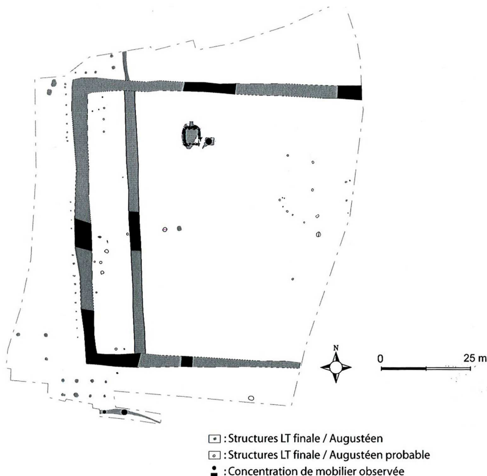
+ Fig. 5. Plan de l'enclos du site du Pré Thomas (Videau 2009).
